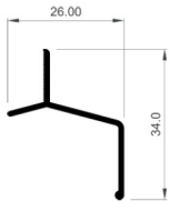
Top rain gutter
